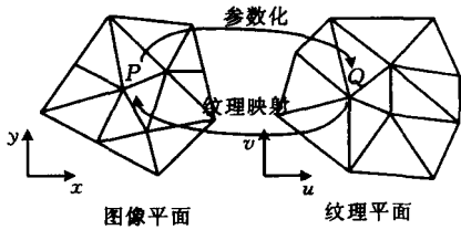
图 3 参数化过程 (借助图像网格点处的法向和投影几何逼近, 我们归结模拟纹理的扭曲形变为一个从二维到二维的参数化优化问题; 求得该参数化结果后, 我们仅仅需要把纹理映射到原始图像的目标区域)
