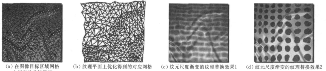
图 5 纹元尺度渐变的纹理替换效果(原始样本纹理尺度均一, 而替换效果的纹元由左上角至右下角逐渐增大)
