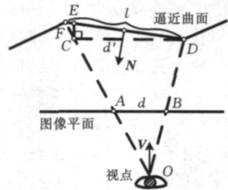
图 2 计算图像区域上边 e(AB) 的真实三维长度 \|FD\| (其中, V 为视线方向, N 为边 e(AB) 的法向在平面 OAB 上的投影, CD \parallel AB 并且 CD \perp CE )
